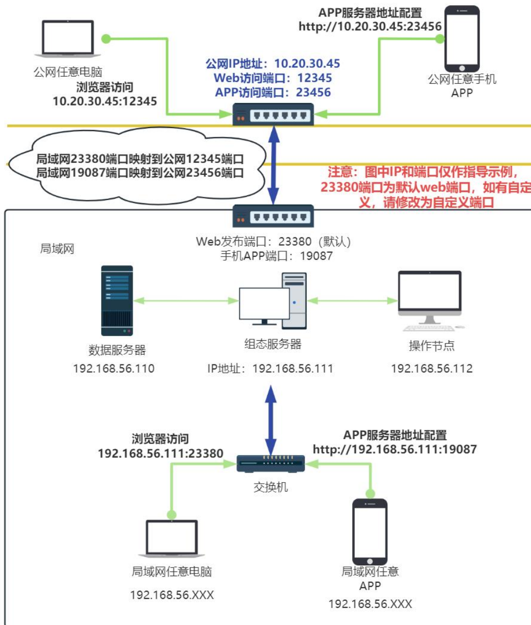
图 1 扩展功能网络架构
