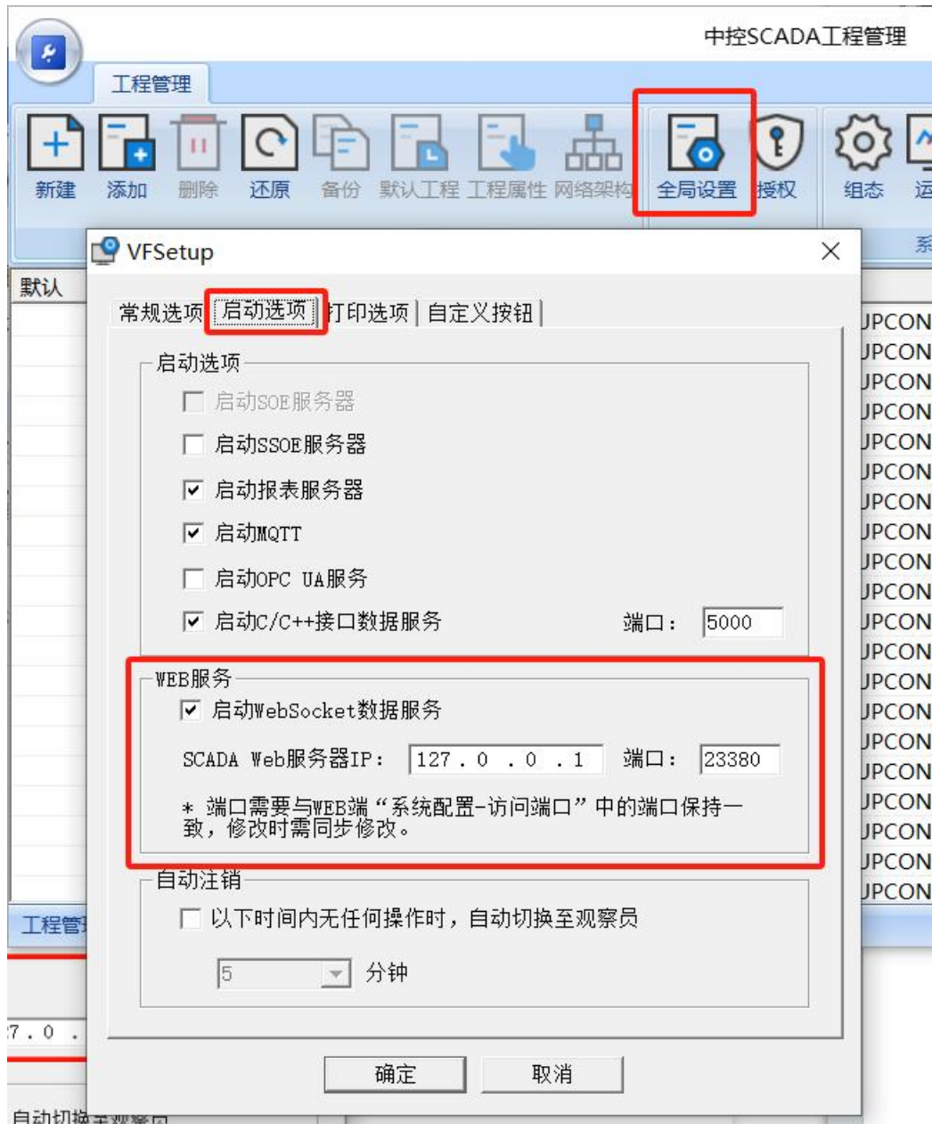
图 3 启动 WebSocket 数据服务
