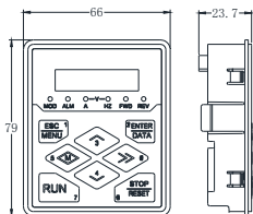
图 2-4 键盘外形尺寸
