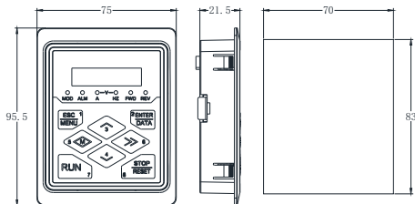
图 2-5 键盘安装盒外形及开孔尺寸
