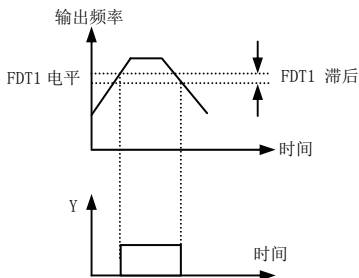
图 7-24 频率水平检测示意图
