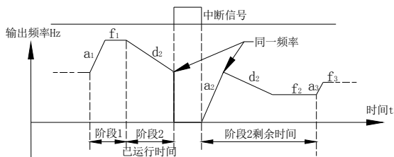
图 7-34 PLC 启动方式 1
