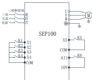
图 7-14 多段速运行接线图
