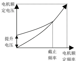
a: 递减转矩曲线转矩提升示意
