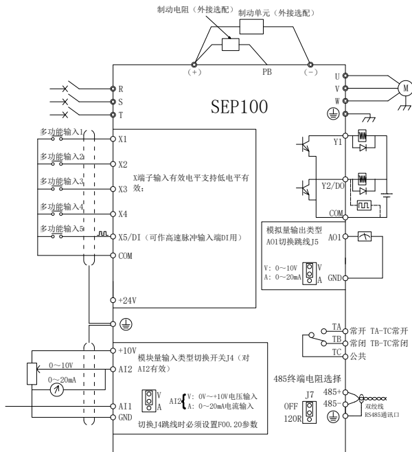
图 3-9 基本配线图
