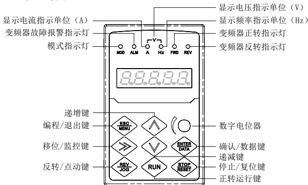
图 C-1 SEP-LED11-D 操作键盘布局图
